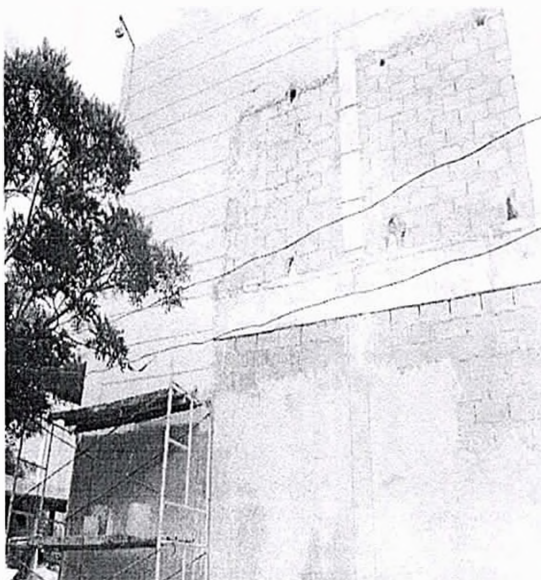
Estructura, mampostería y pañete
