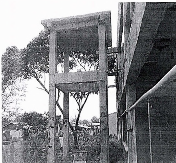
Instalaciones Eléctricas – Estructura para tanque elevado
